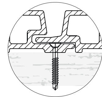
Schroefbevestiging (WEO 60)
